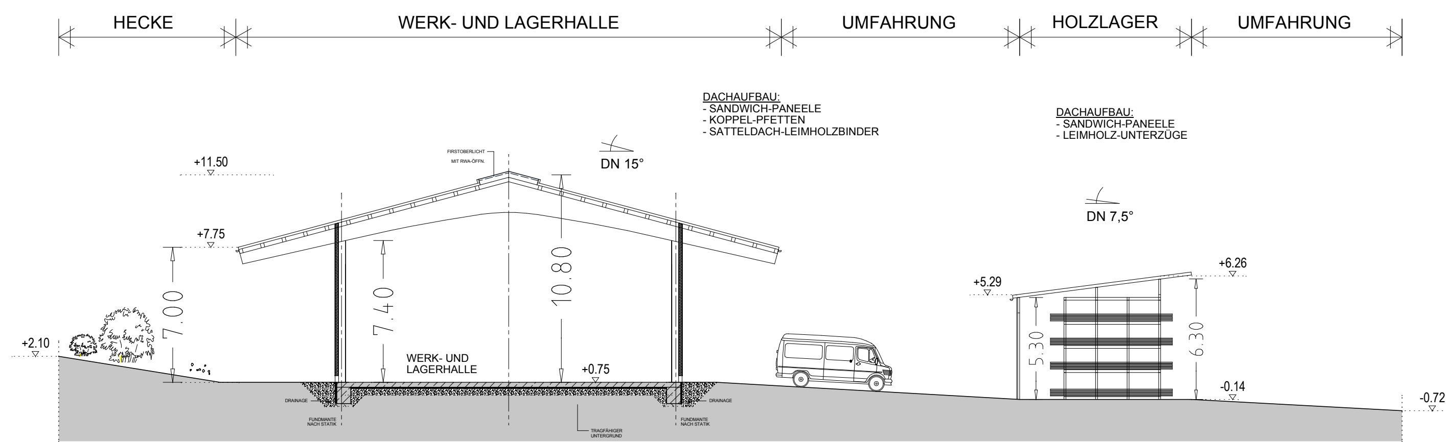
SCHNITTE A-A - M 1:200 WERK- UND LAGERHALLE / HOLZLAGER [ÜBERDACHT]
