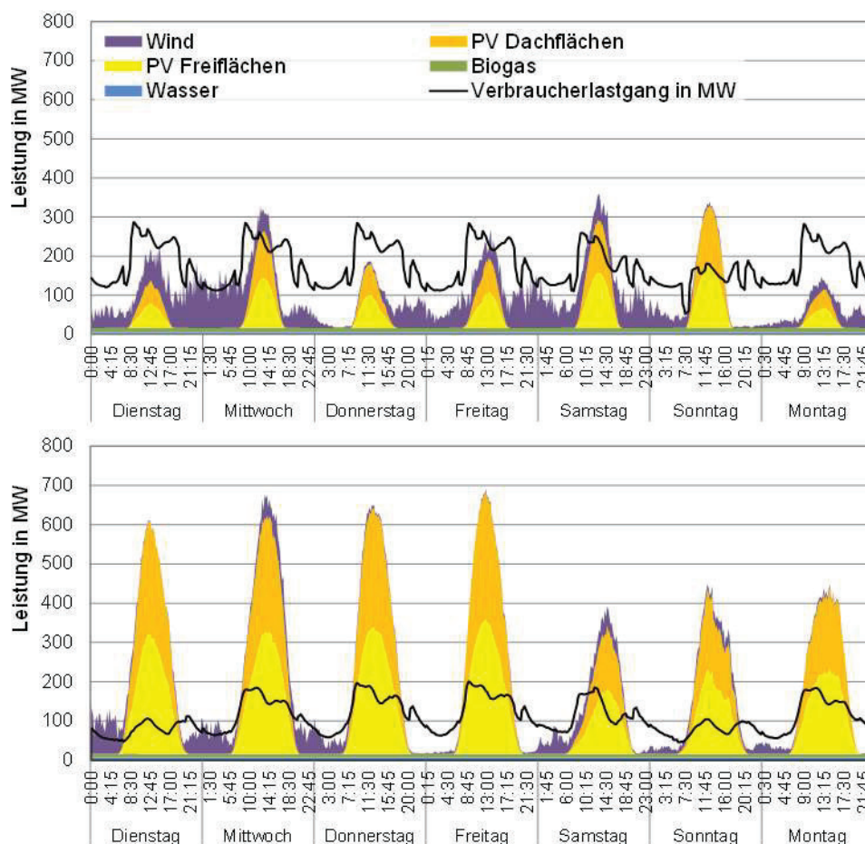
Abbildung 7.4: Strom-Lastganganalyse für das Zieljahr 2024. Oben für den Zeitraum 04. bis 10. Februar, unten für den Zeitraum 01. bis 07. Mai
