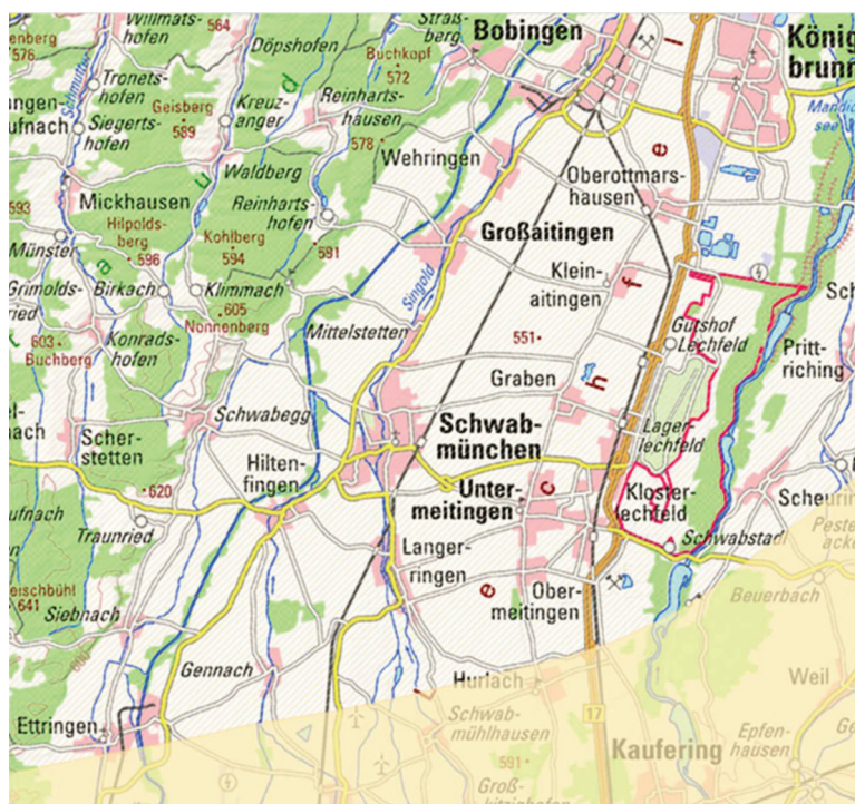
Abbildung 4.7: Eignungsgebiete für hydrothermale Warmegewinnung (LfU, 2024 b) Günstige geologische Verhältnisse für hydrothermale Warmegewinnung Weniger günstige Verhältnisse für hydrothermale Warmegewinnung (i.d.R. zusätzlicher Wärmepumpeinsatz erforderlich)
