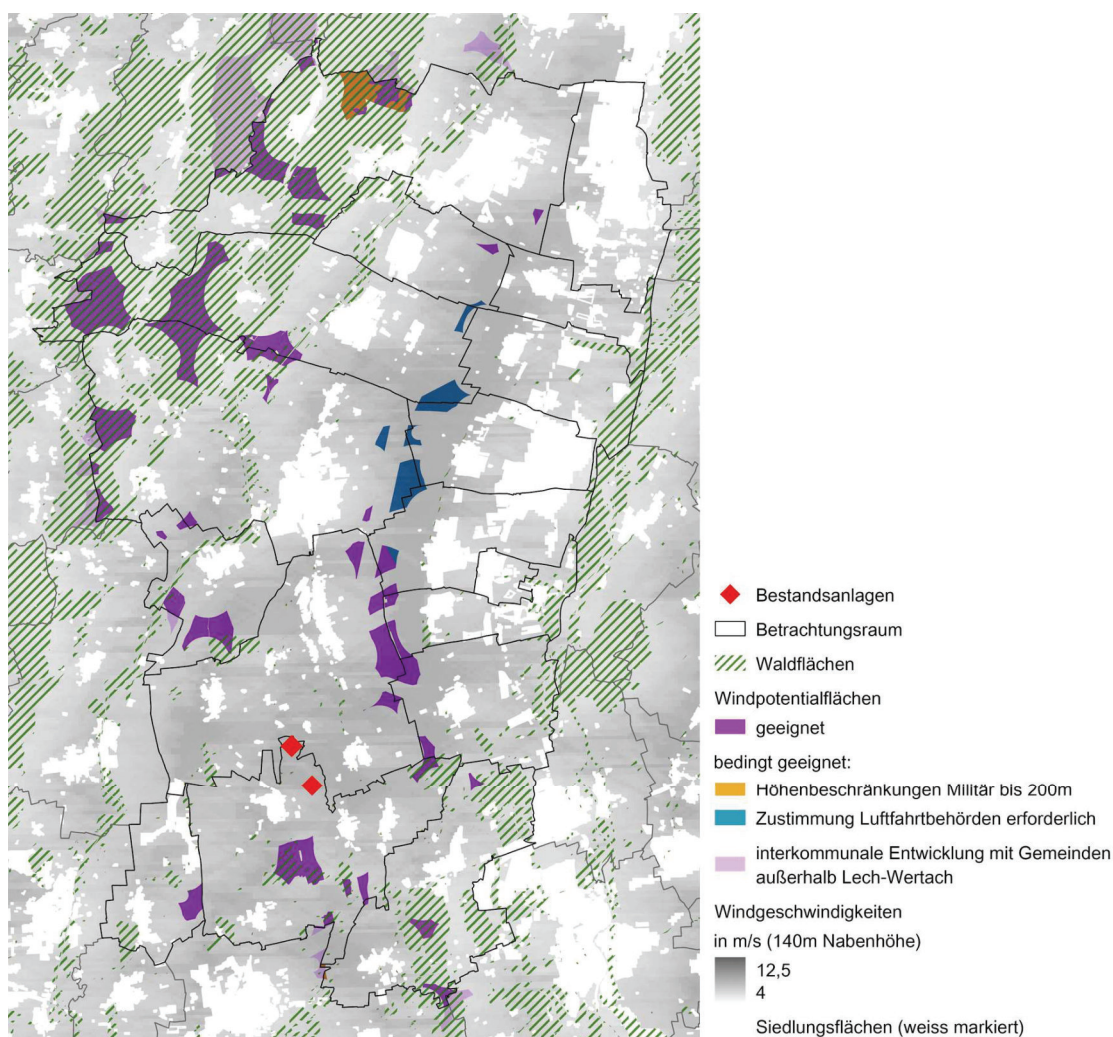
Abbildung 4.3: Windpotentialflächen und Bestandsanlagen im Betrachtungsraum
