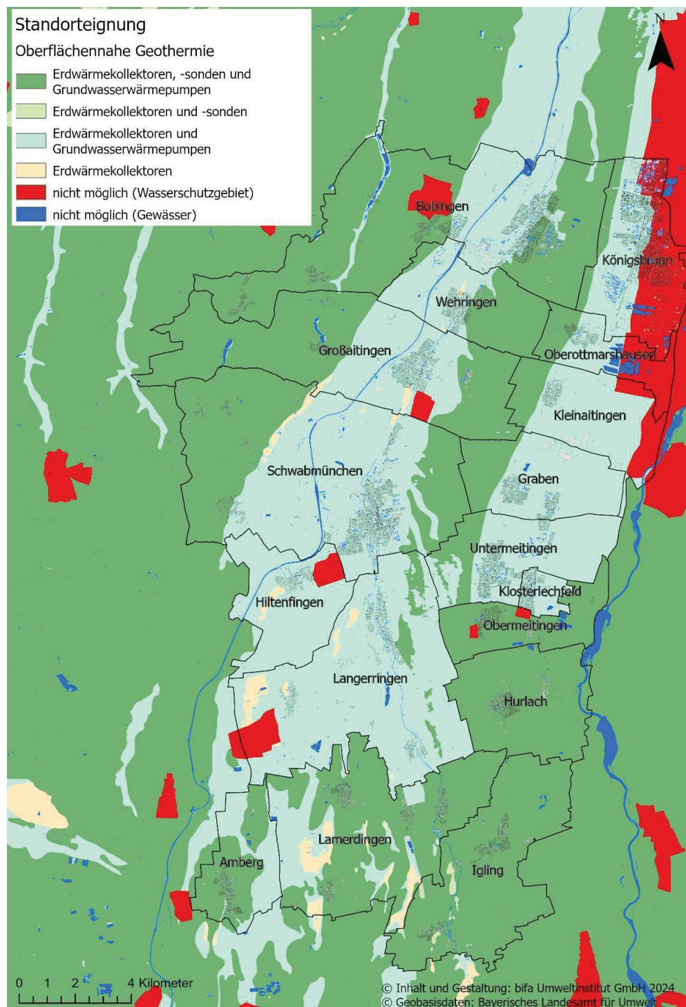
Abbildung 4.6: Eignungsgebiete für die Nutzung unterschiedlicher oberflächennaher Geothermiesysteme
