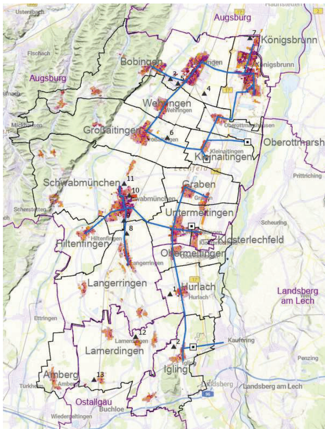
Abbildung 7.12: Wärmenetztrassen (blau) verbinden potentielle geothermische Förderstandorte (schwarz-weiße Punktmarkierung) mit Abnahmezentren. Abgebildet: Zweiteilige Versorgung (Nord und Süd).
