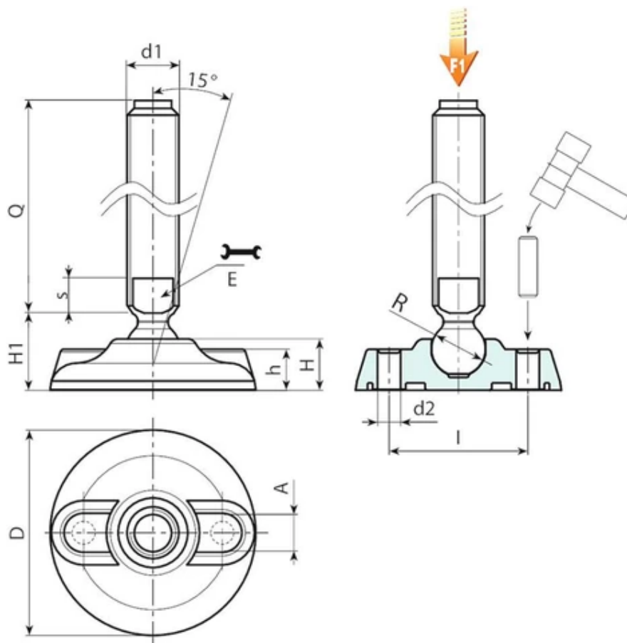
Версия P913: Опора со стержнем типа В (с фрезерованной лыской под ключ) и шаровой головкой 15
