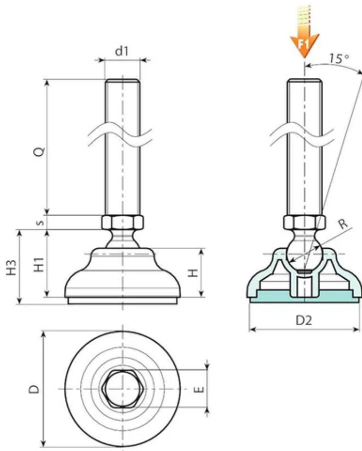
Версия P901: Опора со стержнем типа А (шестигранное основание), шаровая головка 12,4, противоскользящее основание из термопластичной резины SBS
