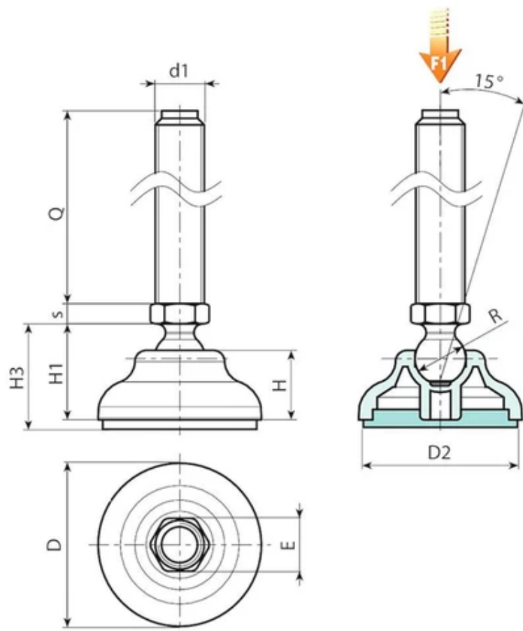
Версия P908: Опора со стержнем типа А (шестигранное основание), шаровая головка 15, противоскользящее основание из термопластичной резины SBS
