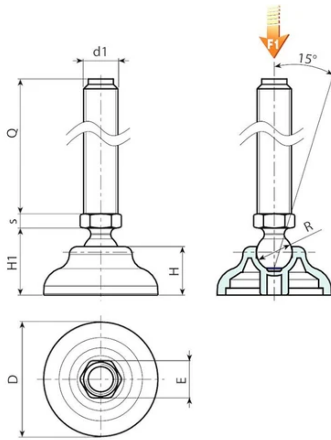
Versão P905: Pé de apoio com perno tipo A (com hexágono) e esfera 15
