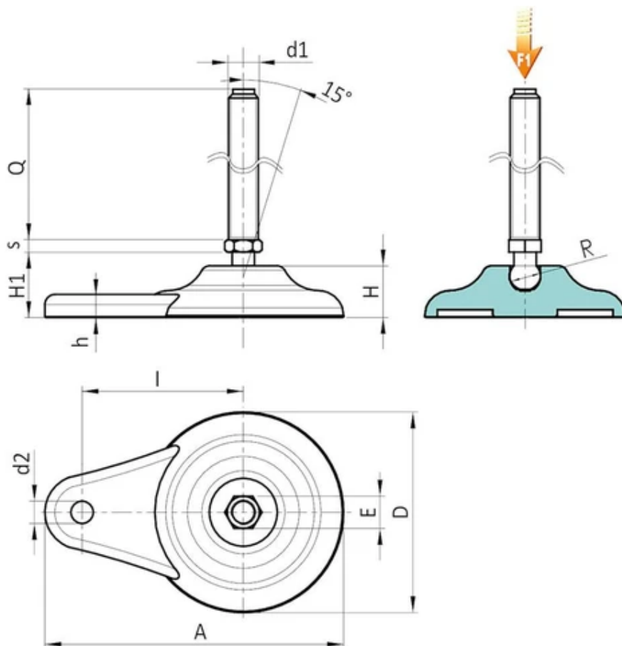
P700 változat: Csepp alakú rögzítő láb talajrögzítéssel - A típusú szárral - (hatszögletű talppal) és 12.5 golyóval
