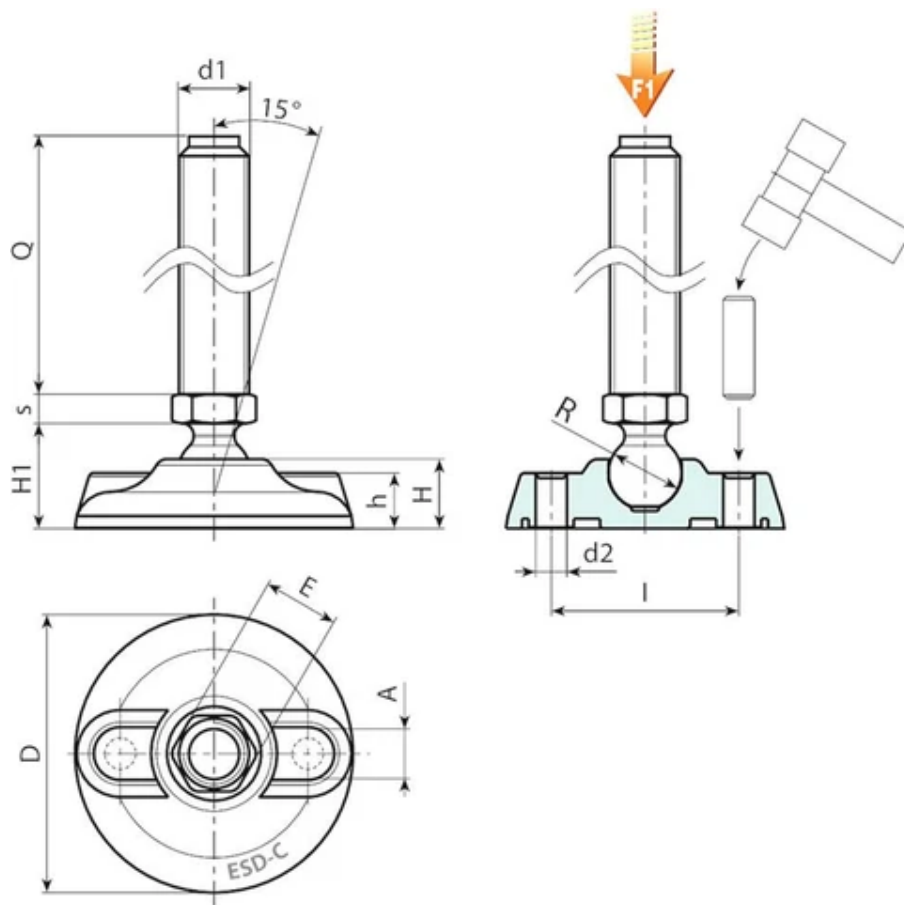
P902ESD változat: Rögzítő láb A típusú szárral (hatszögletű talppal) és 15 golyóval
