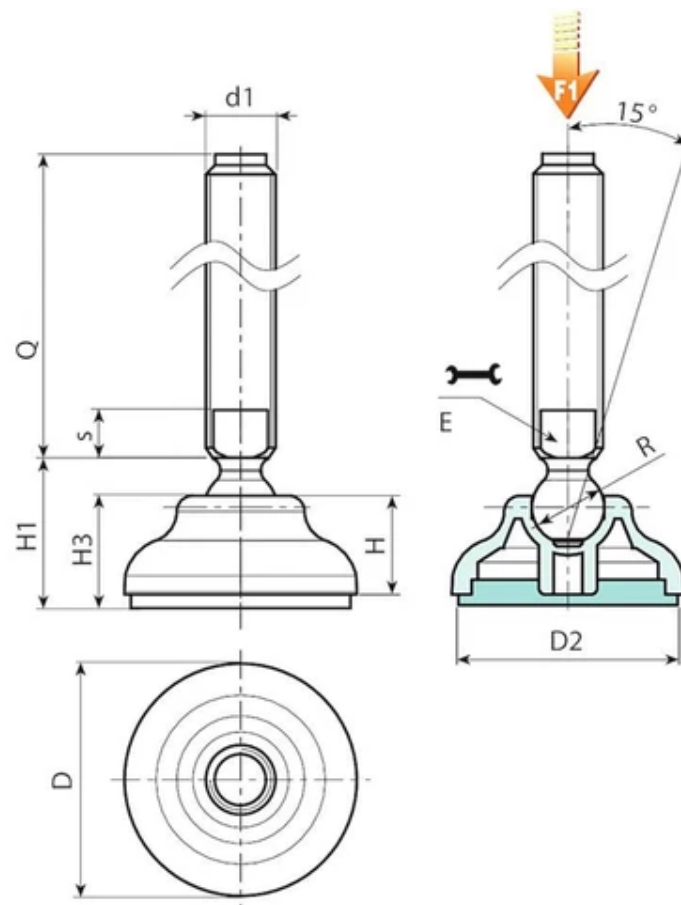
P910 változat: Rögzítőláb B típusú szárral (hornyolt foglalattal a csavarkulcshoz) és 15 golyó - SBS csúszásmentes talppal
