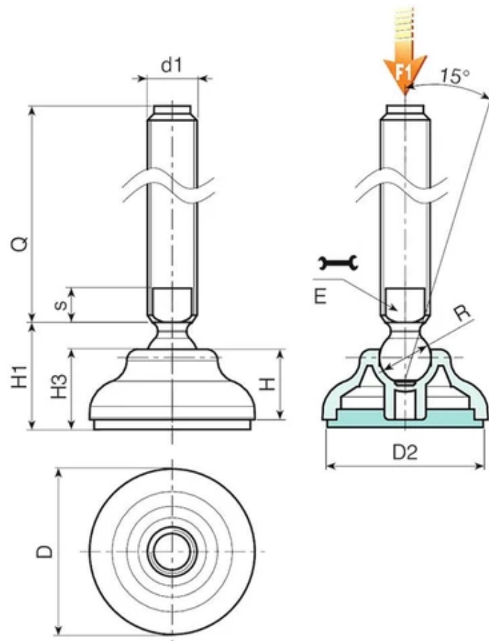
Versio P909: Tukijalka, B-tyyppinen varsi (avainpesä jyrskyty) ja pallo 12,4 - luistamisenesto SBS-kumia
