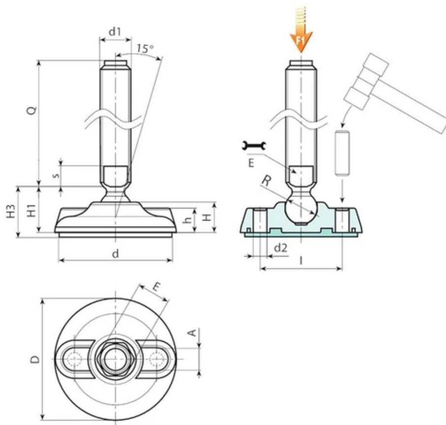
Versio P917: Tukijalka, B-tyyppinen varsi (avainpesä jyrsitty) ja pallo 15 - luistamisenesto SBS-kumia
