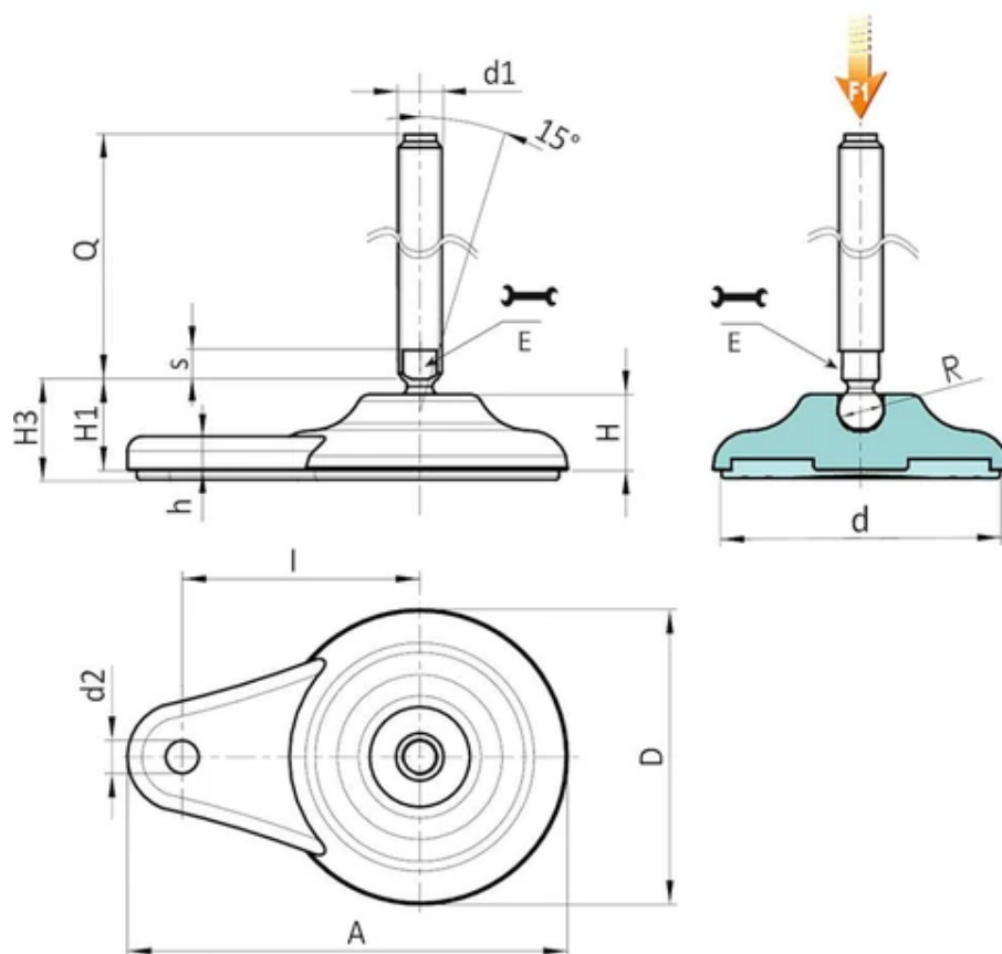
Versión P707: Pie de apoyo con fijación lateral, perno tipo B (alojamiento fresado para llave) y bola 15 - con base antideslizante de SBS
