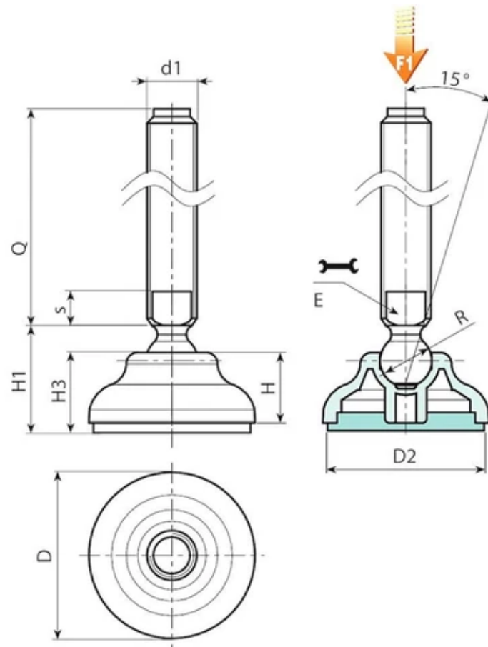
Ausführung P910: Gelenkfuß mit Verstellspindel Typ B (mit Aufnahme für Gabelschlüssel) und Kugel 15 - mit rutschfester Gummiauflage aus SBS
