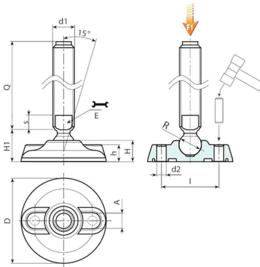
Ausführung P913: Gelenkfuß mit Verstellspindel Typ B (mit Aufnahme für Gabelschlüssel) und Kugel 15
