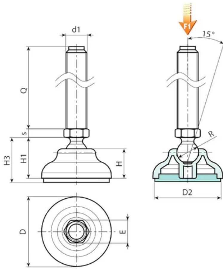
Ausführung P908: Gelenkfuß mit Verstellspindel Typ A (mit Aufnahme für Gabelschlüssel)-Kugel 15-mit rutschfester Gummiauflage aus SBS
