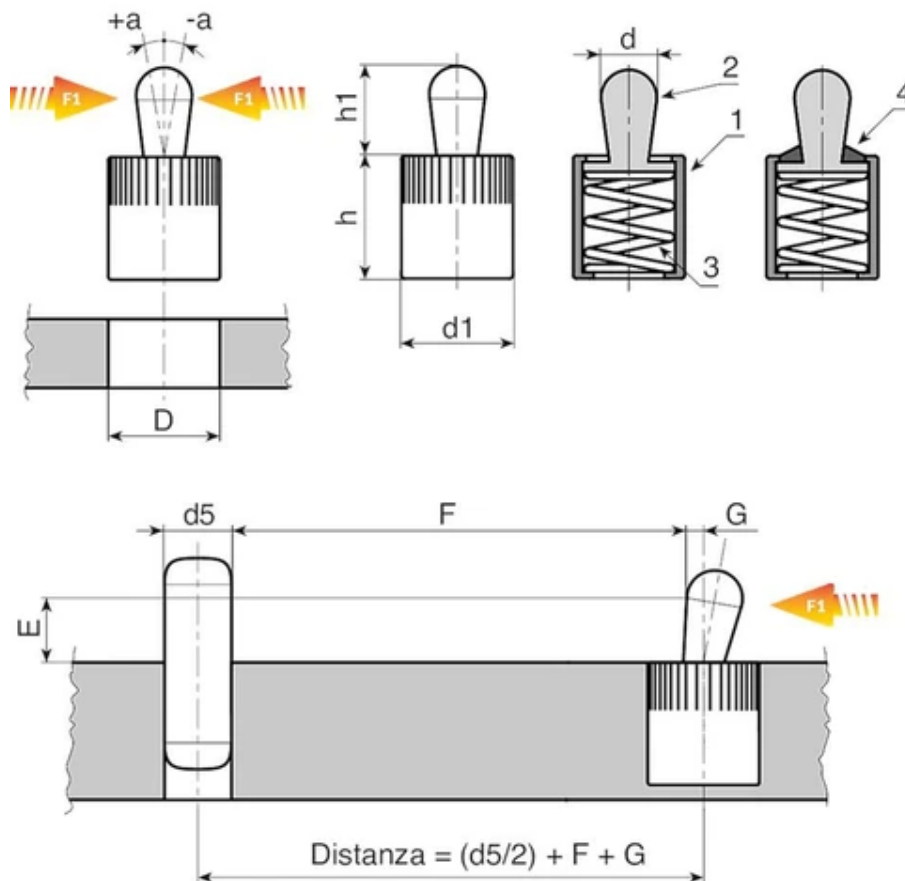
Versie W615: Zij-aandrukstuk met drukpen in POM en pakking
