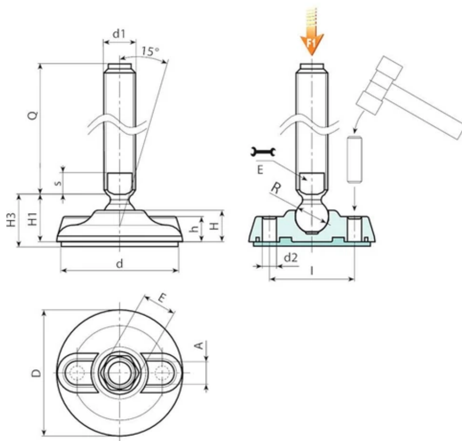
Version P918: Støttefod med skafttype B (fræset nøglesæde) og kugle 24 - med skridsikring i SBS
