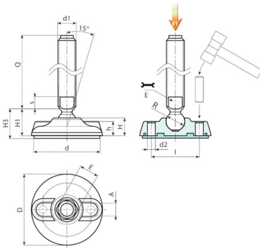
Wersja P917: Stopka podporowa z trzpieniem typu B (z frezowanym gniazdem pod klucz) i kulką 15 - z podstawą antypoślizgową z SBS
