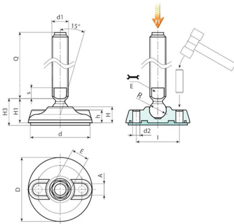
P917 változat: Rögzítőláb B típusú szárral (hornyolt foglalattal a csavarkulcshoz) és 15 golyó - SBS csúszásmentes talppal
