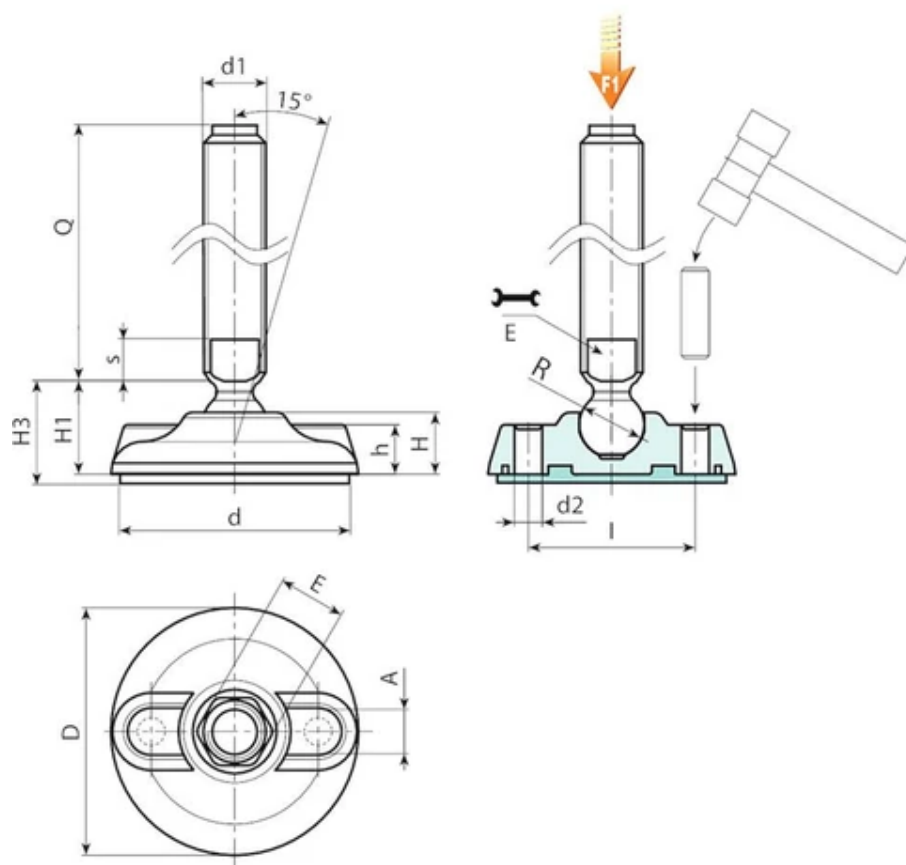
Versión P917: Pie de apoyo con perno tipo B (alojamiento fresado para llave) y bola 15 - con base antideslizante de SBS
