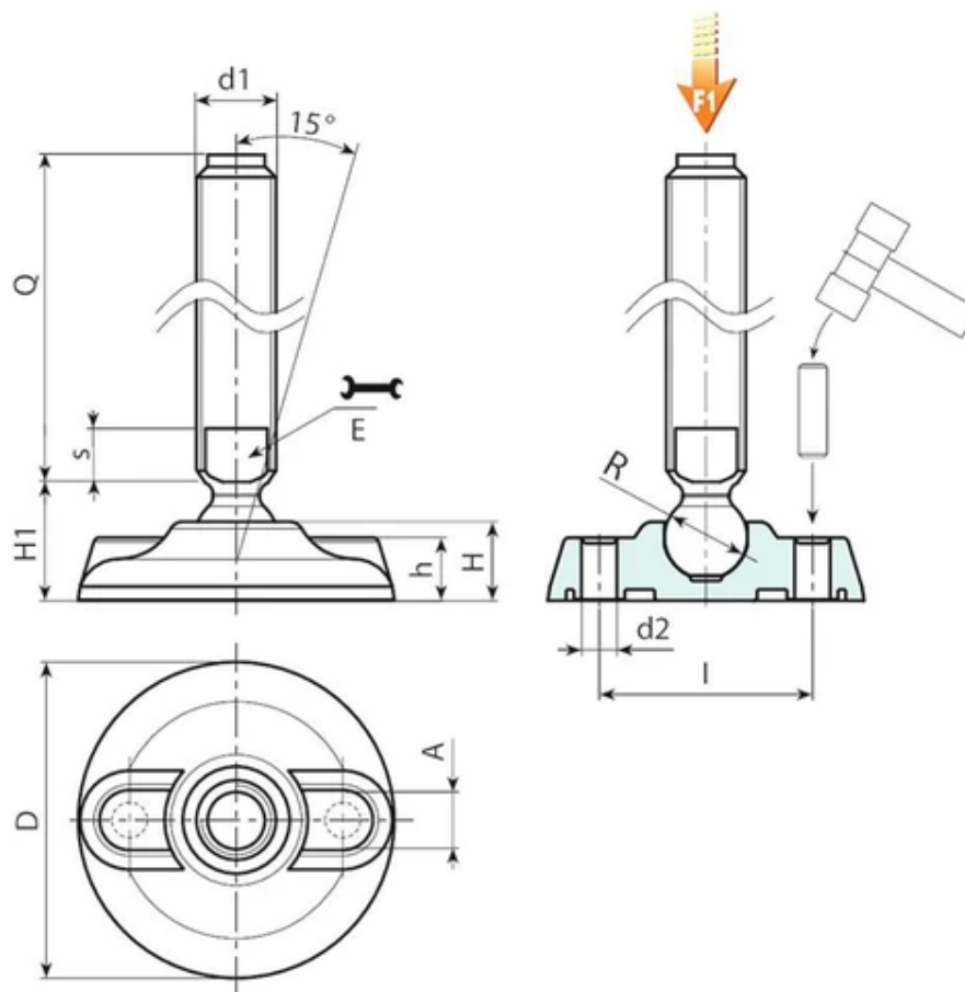
P914 változat: Rögzítőláb B típusú szárral (hornyolt foglalatnál a csavarkulcshoz) és 24 golyó
