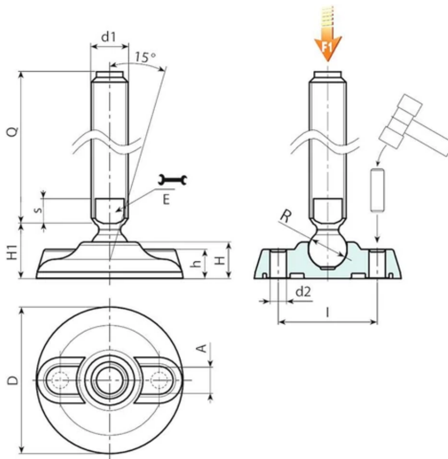
Version P914 : Pied d'appui avec tige de type B (logement pour clé fraisé) et bille 24
