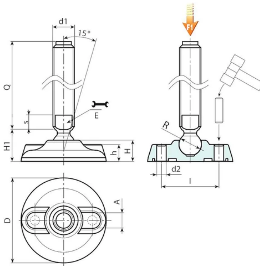
Версия P913: Опора со стержнем типа В (с фрезерованной лыской под ключ) и шаровой головкой 15
