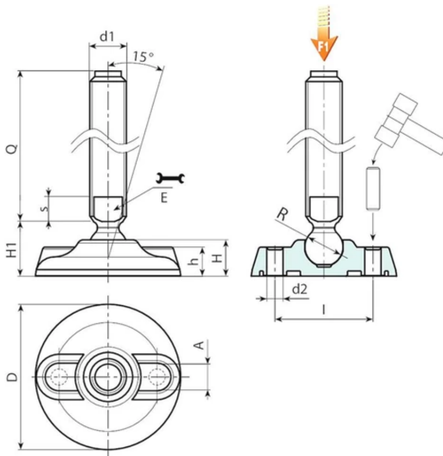
P913 változat: Rögzítőláb B típusú szárral (hornyolt foglalattal a csavarkulcshoz) és 15 golyó
