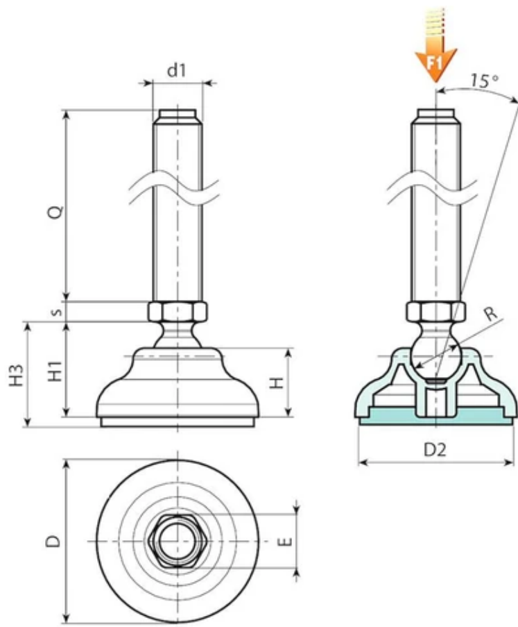
Versão P908: Pé de apoio com perno tipo A (base hexagonal) e esfera 15 - com antiderrapante em SBS
