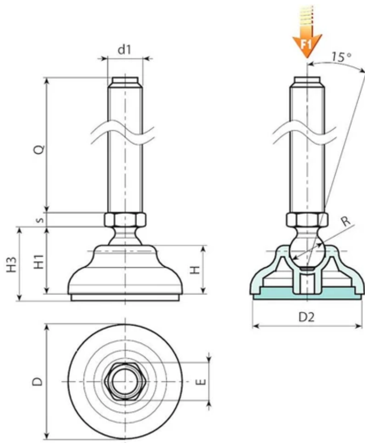
P908 változat: Rögzítőláb A típusú szárral (hatszögletű talppal) és 15 golyóval - SBS csúszásmentes talppal
