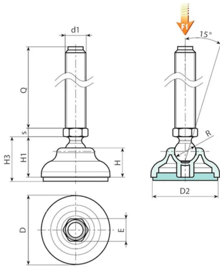
Version P908: Støttefod med skafttype A (sekskantet bund) og kugle 15 - med skridsikring i SBS
