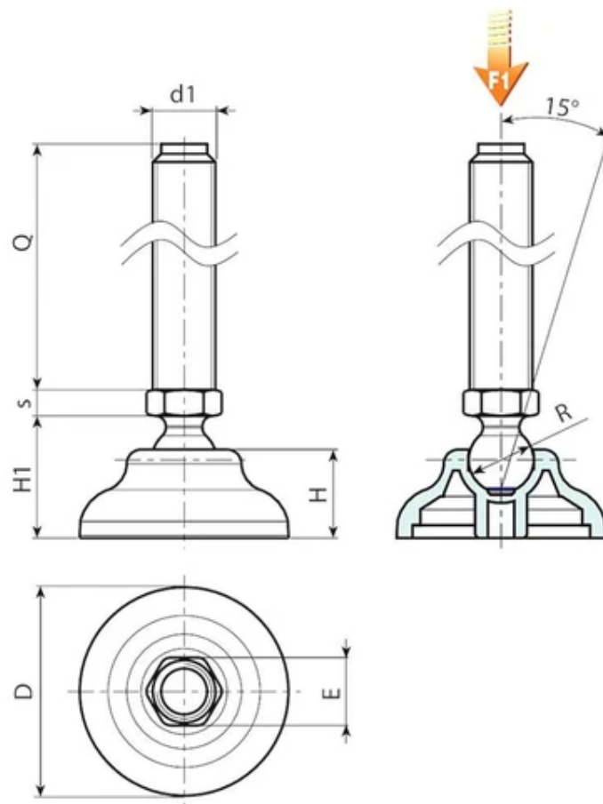
P905 változat: Rögzítőláb A típusú szárral (hatszögletű talppal) és 15 golyóval
