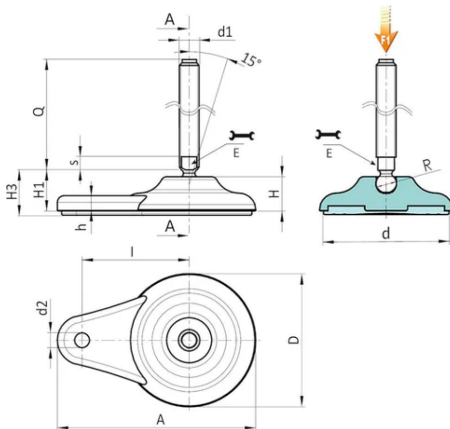
Ausführung P705: Gelenkfuß mit Verstellspindel Typ B - aus PA - (mit Aufnahme für Gabelschlüssel) und Kugel 12,5 - mit rutschfester Gummiauflage aus SBS
