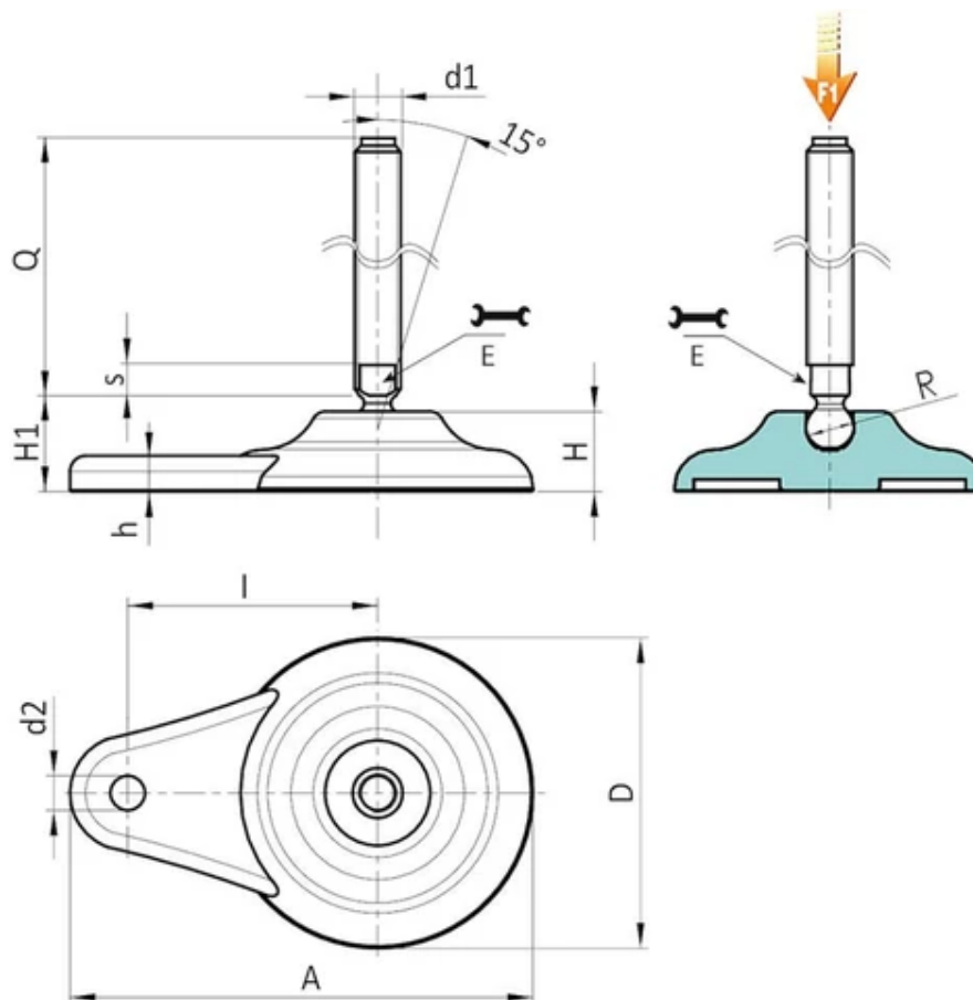
P704 változat: Csepp alakú rögzítőláb talajrögzítéssel - B típusú szárral (hatszögletű talppal a csavarkulcshoz) és 12.5 golyóval
