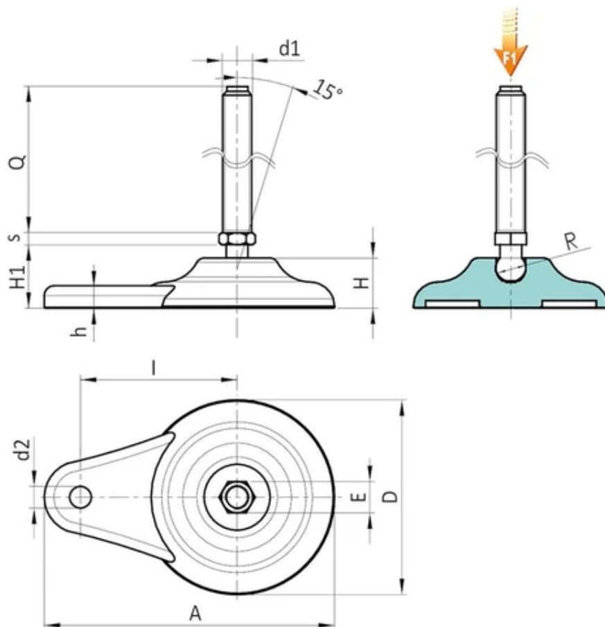
Версия P700: Опора с боковым креплением, со стержнем типа А (с шестигранником) и шаровой головкой 12,5
